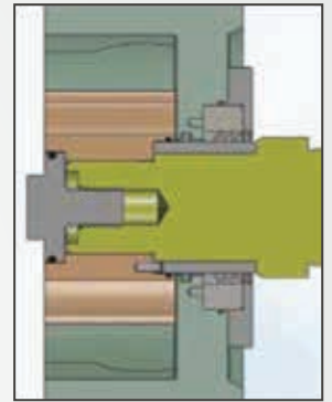
Sello de triple labio
